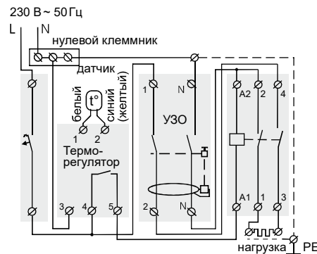
Схема 2. Подключение через магнитный пускатель
