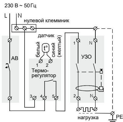
Схема 1. Подключение АВ и УЗО
